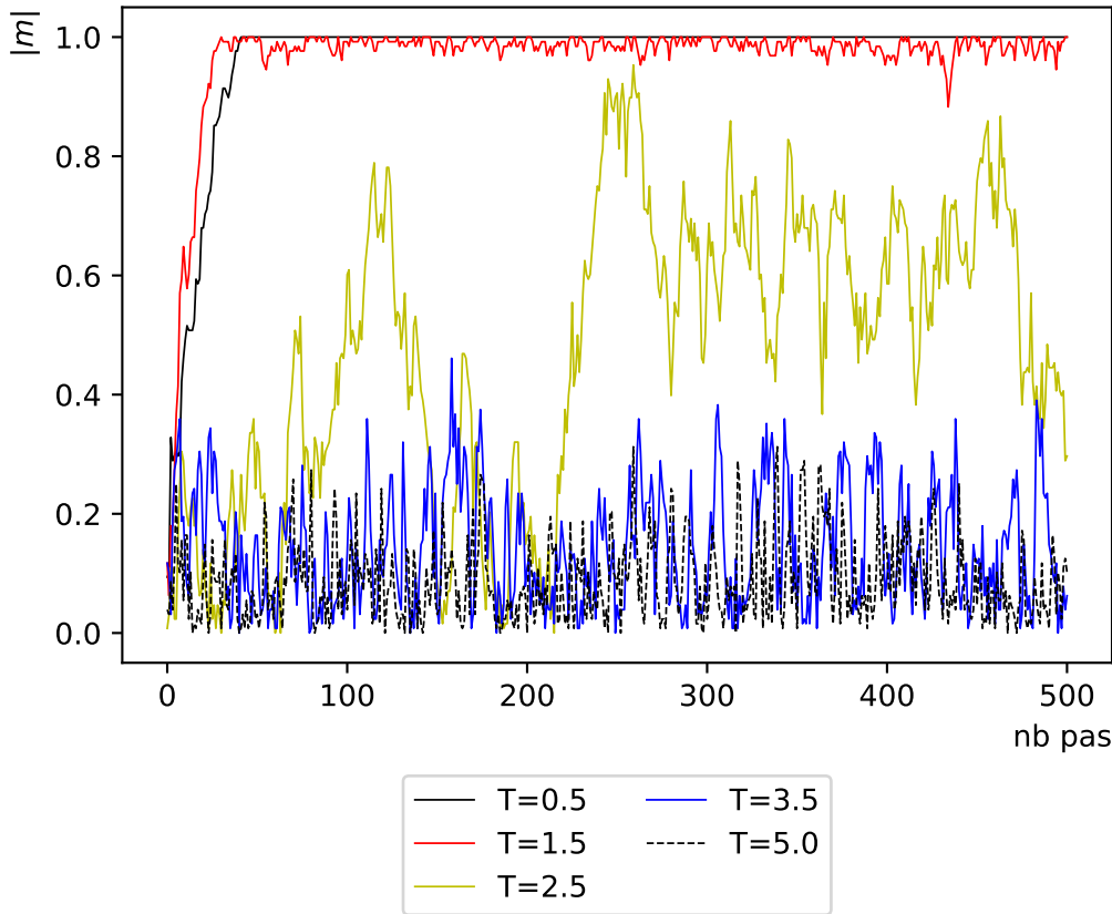
Evolution de l'aimantation sur 500 pas de Monte Carlo, N=16
